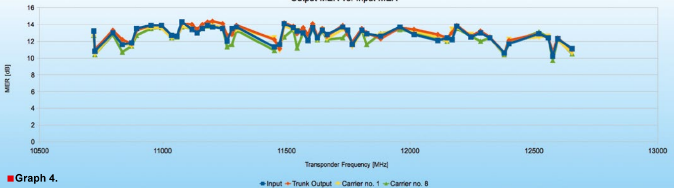
SUS 4481 F Output MER vs. Input MER
