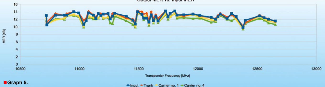
SUS 5541 NFA Output MER vs. Input MER
